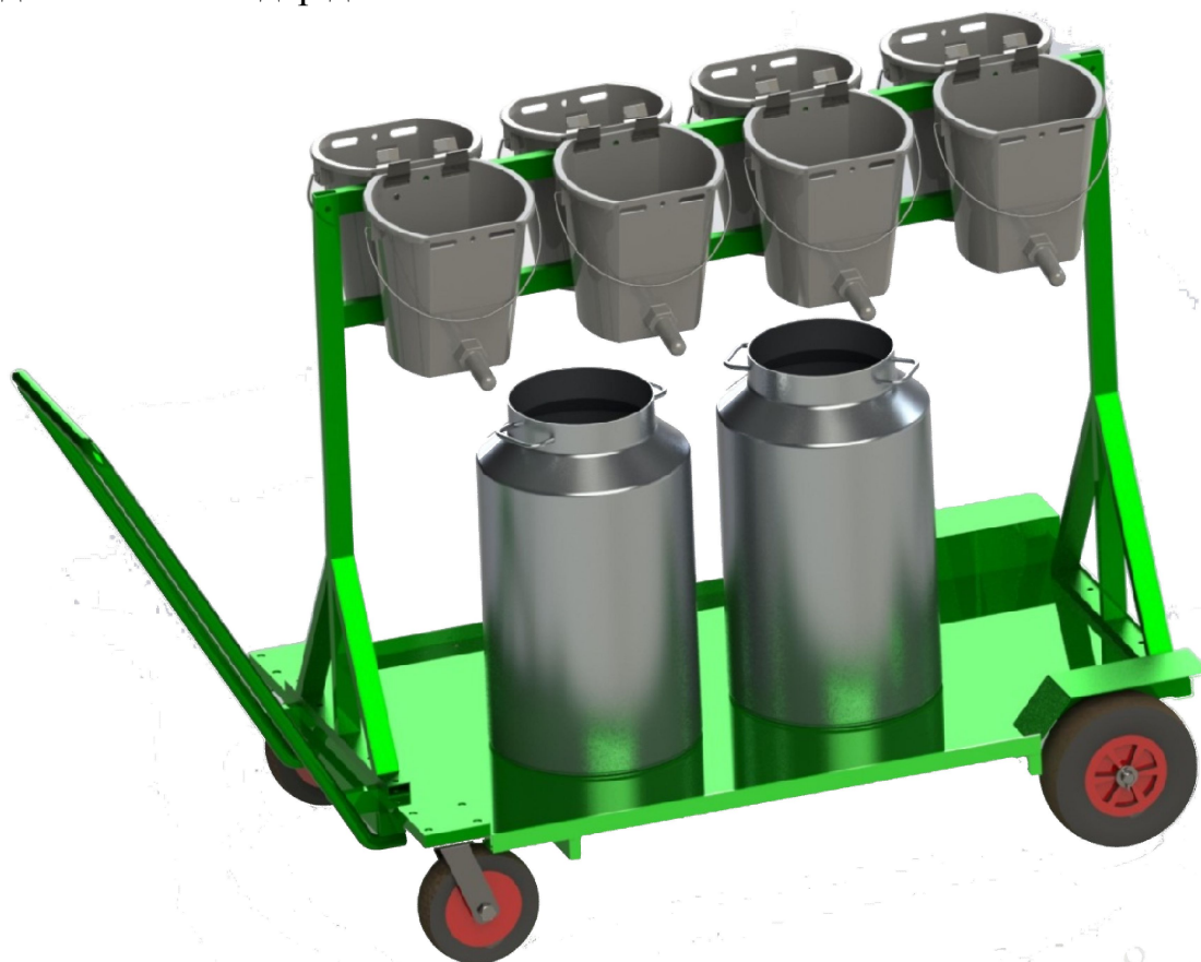
Рис 1. - Тележка для транспортировки бидонов ТТВ-1
